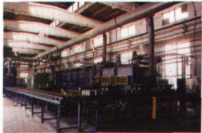
连续式渗碳自动线
