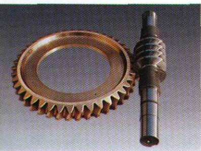
蜗轮副
