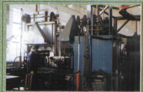
LSX22 辐射管式连续渗碳淬火回火清洗自动生产线
