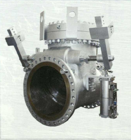
高排及抽汽逆止阀
