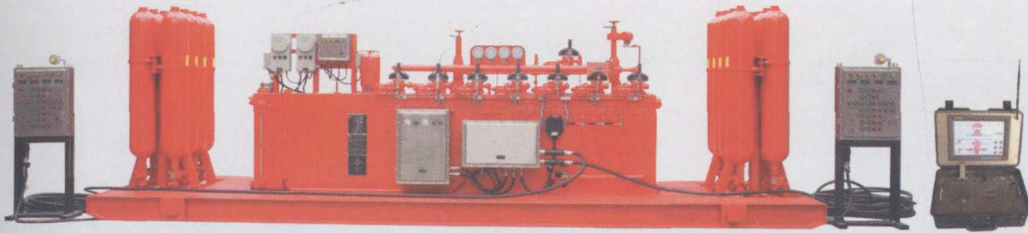
FKWDQ1280-7无线遥控防喷器控制装置
