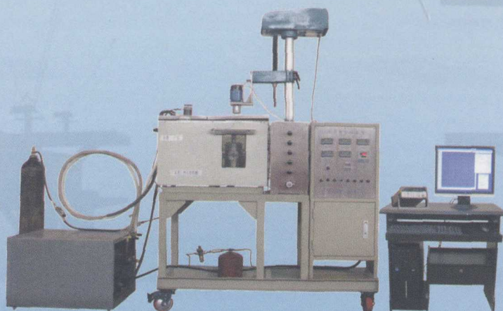
可视化水合物（可燃冰）形成装置
