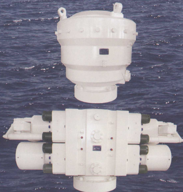
F48-105 水下防喷器
