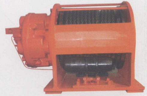
HW/1600型液压旋转猫头
