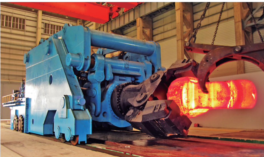
超大夹持力和夹持力矩 (300t和750t·m)全液压锻造操作机
