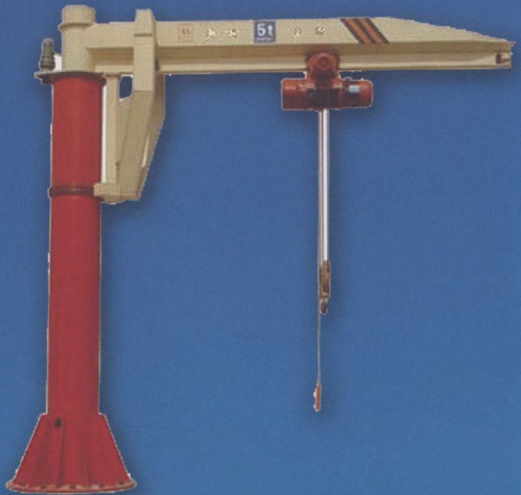
悬臂起重机
