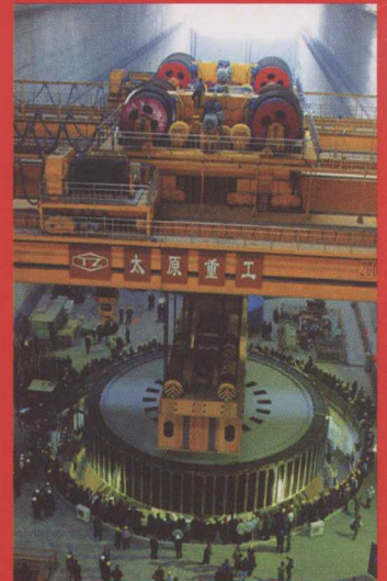
◆ 三峡电站1200t桥式起重机
