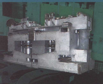
▲液压振动装置
