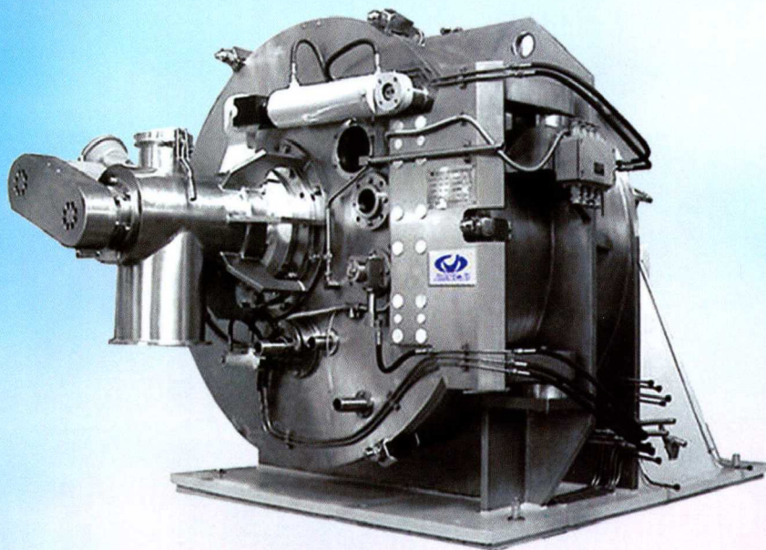
GKH卧式虹吸刮刀卸料离心机
