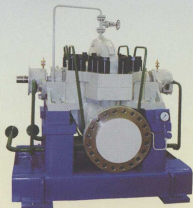
配套1 000MW核电机组FA1D低压安注喷淋泵
