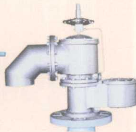
先导式呼吸阀
