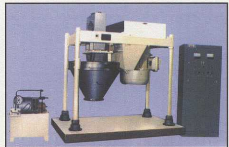
LZM系列针型冲击磨, 淀粉行业物料粉碎的最佳细磨设备
