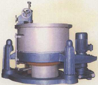
SG 系列离心机 三足式手动刮刀下部卸料
