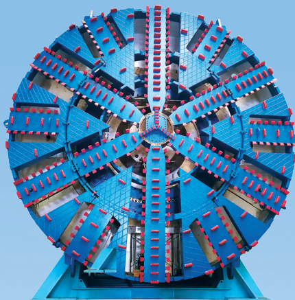
孟加拉卡纳普里河底隧道工程 直径 12.12m 气垫式泥水平衡盾构机
