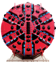
福州地铁 Φ 6460mm 复合式土压盾构机
