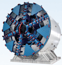
南昌地铁 Φ 6260mm 软土盾构机
