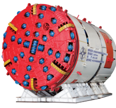
深圳地铁 Φ 6470mm 双护盾 TBM
