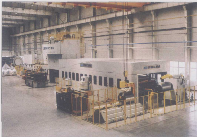
● 由1台J39C—500A型闭式四点单动落料压力机和开卷、校平、送料、磁性码垛等自动化装置组成的ZSK—3×1850开卷校平落料自动线（安装在长城汽车股份有限公司）
