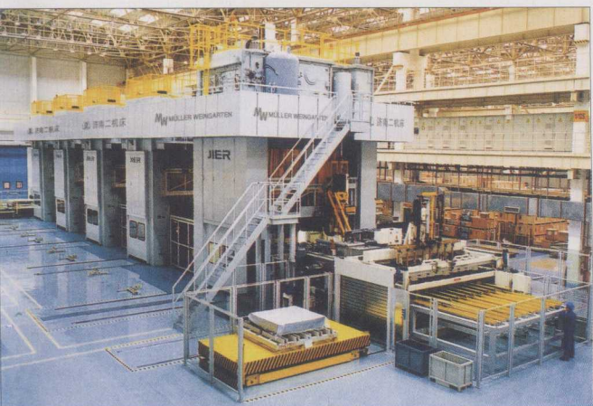
● 由1台LS4-2000型、4台JB39-1000B型闭式四点单动压力机和冲压自动化系统组成的大型自动化冲压生产线(安装在上海通用东岳汽车有限公司)
