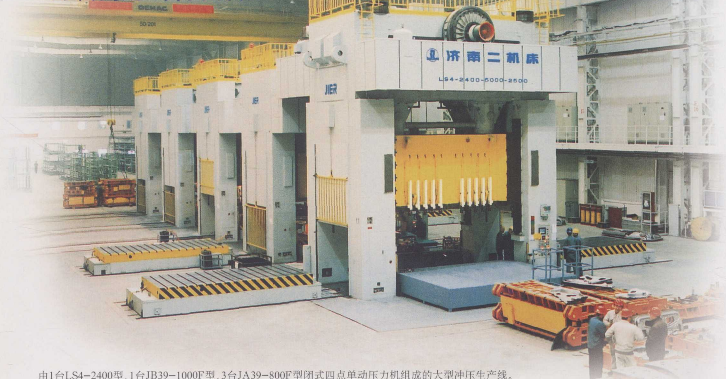
由1台LS4-2400型、1台JB39-1000F型、3台JA39-800F型闭式四点单动压力机组成的大型冲压生产线。
