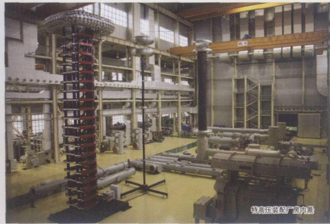
ZF27-1100 GIS投入商业运行的特高压线路晋东南变电站
