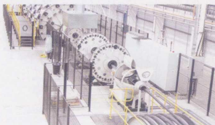
■ KJY摇篮型钢丝绳铠装机
