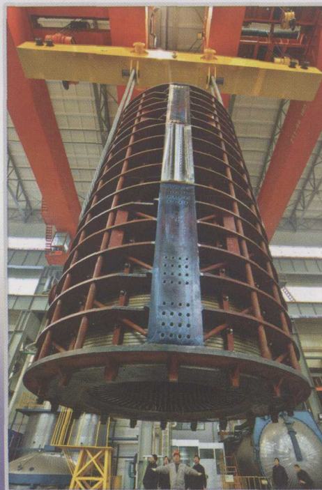
起吊350MW空冷发电机定子
