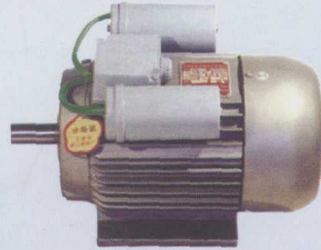
YL系列(H71-100)双值电容单相异步电动机
