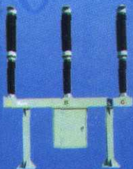
LW41-126型 户外高压SF6柱式断路器
