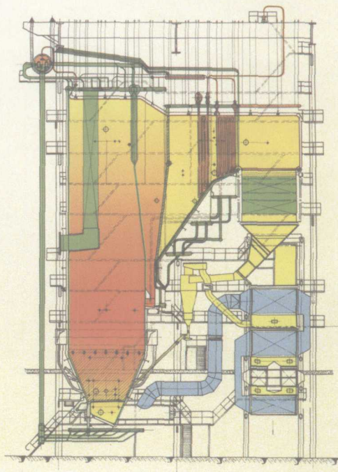
220t/h 循环流化床锅炉
