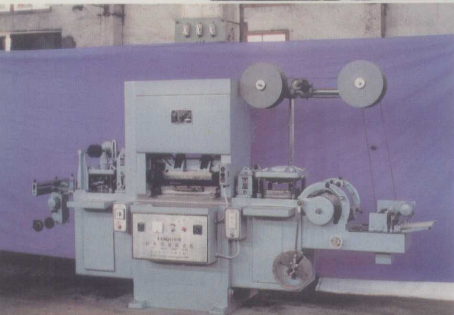
湖北省宜昌印刷机械厂生产的 新一代全功能 LYBG4180 型自动 标签印制联动机
