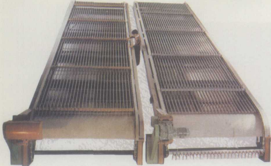
山东省水电设备厂生产的HQ 型回转式清污机
