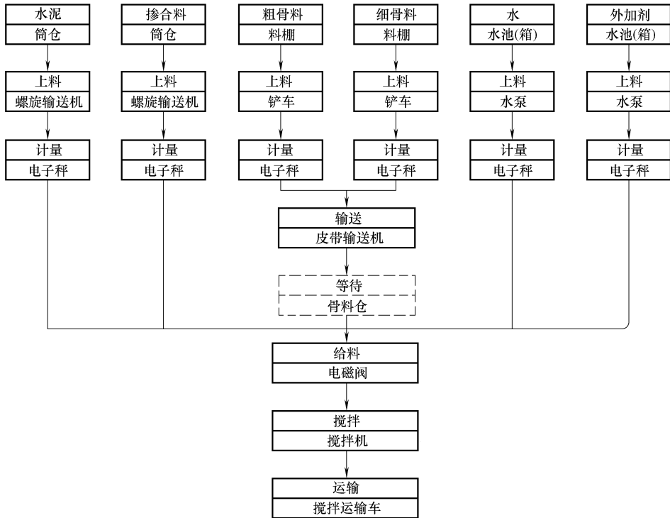
图 1-1 预拌混凝土生产工艺流程
