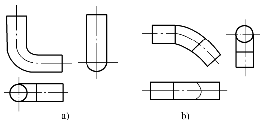
图 1-6 90^\circ 弯头和 45^\circ 弯头双线图
