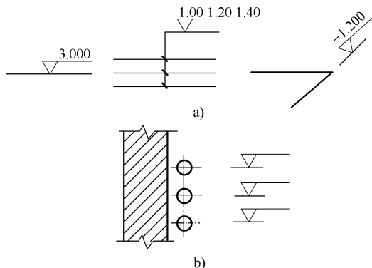
图 1-3 标高符号及注法
