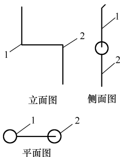
图 1-8 来回弯的三面投影图
