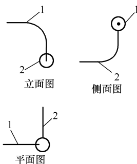
图 1-9 摇头弯的三面投影图
