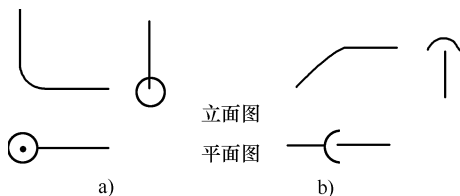
图 1-7 弯头单线图
