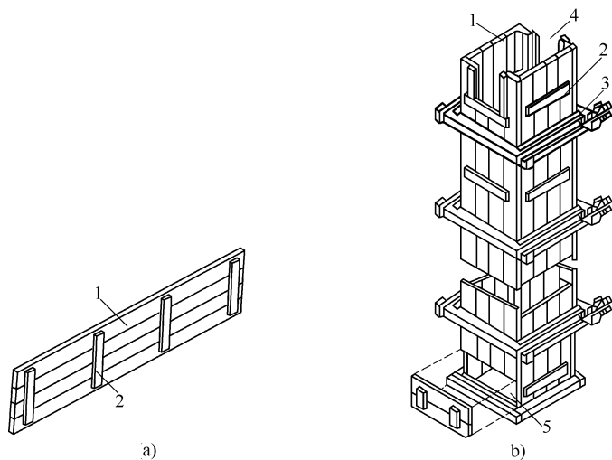
图 1-5 木模板
