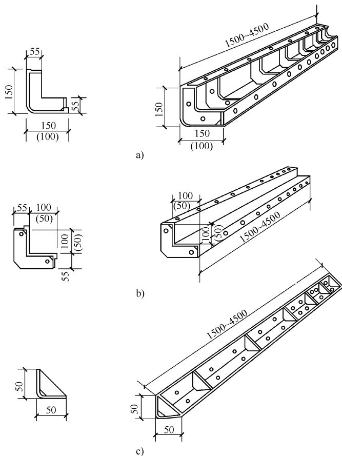
图 1-3 转角模板
