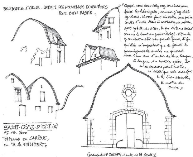
图 1-2 设计手绘图(二)
