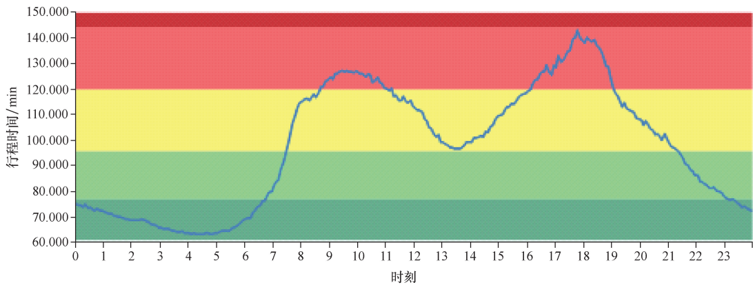
彩图 4 图 3-18 考虑预留时间时行程时间分时变化图
