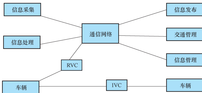
图 1-1 ITS 通信系统示意图
