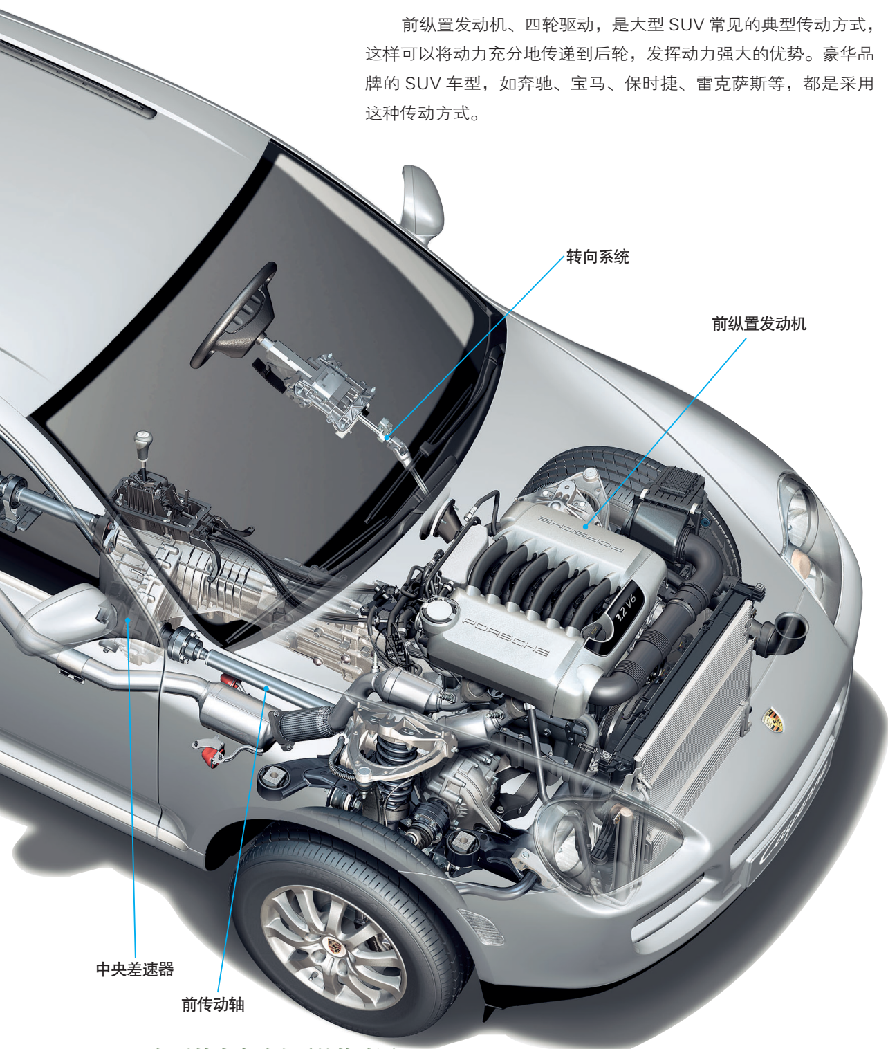
保时捷卡宴动力系统构造图
