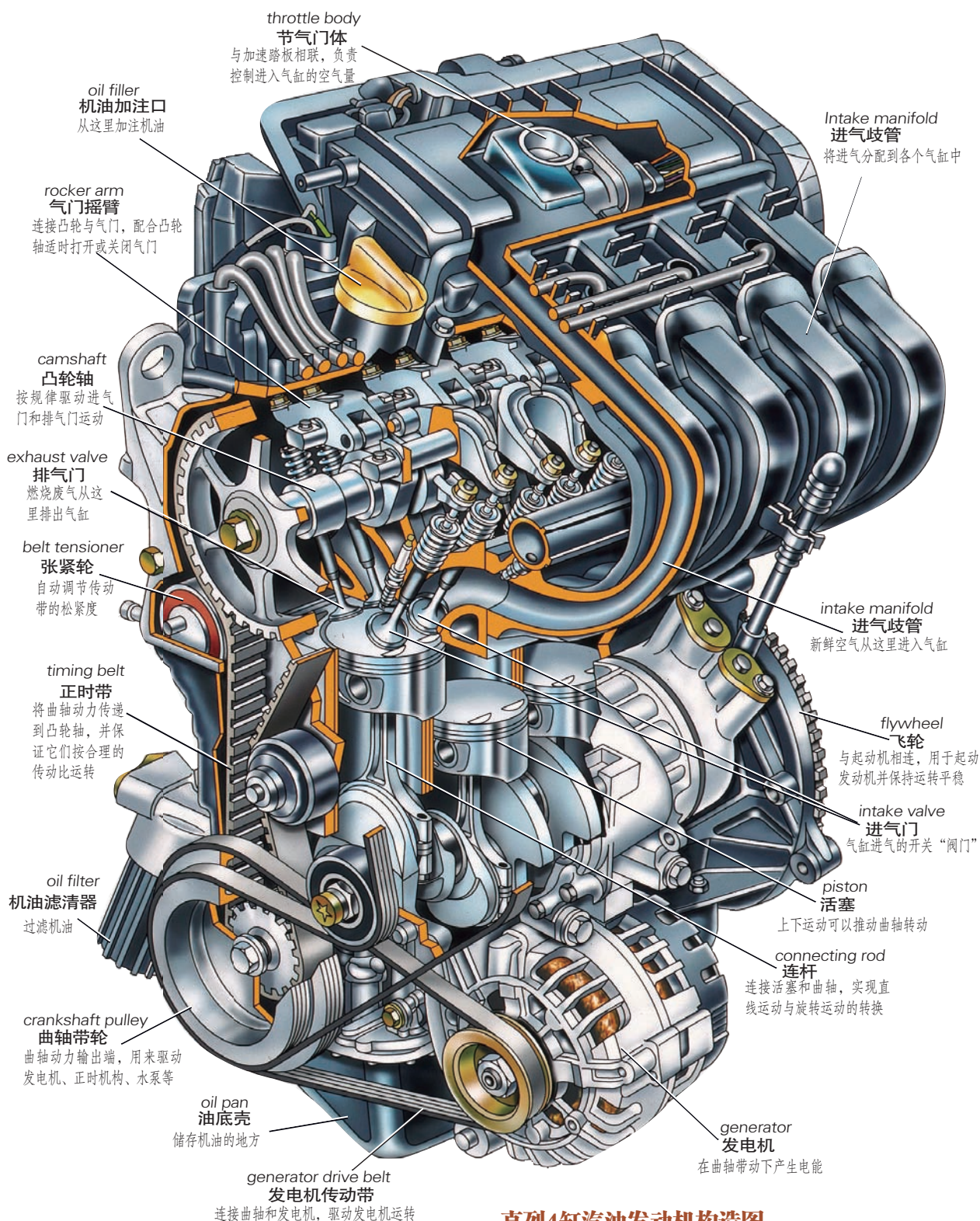
直列4缸汽油发动机构造图
