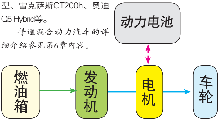
普通混合动力汽车原理示意图
