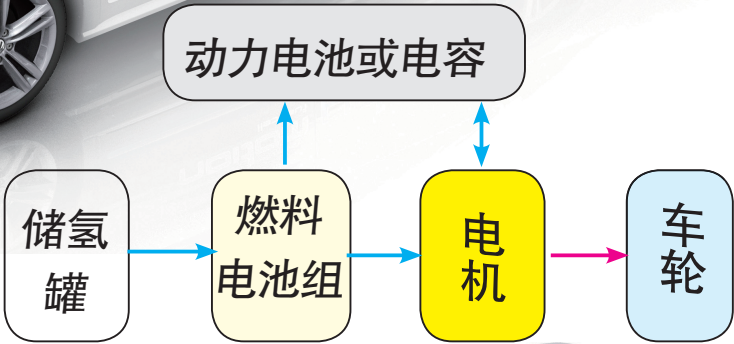
燃料电池汽车构造示意图
