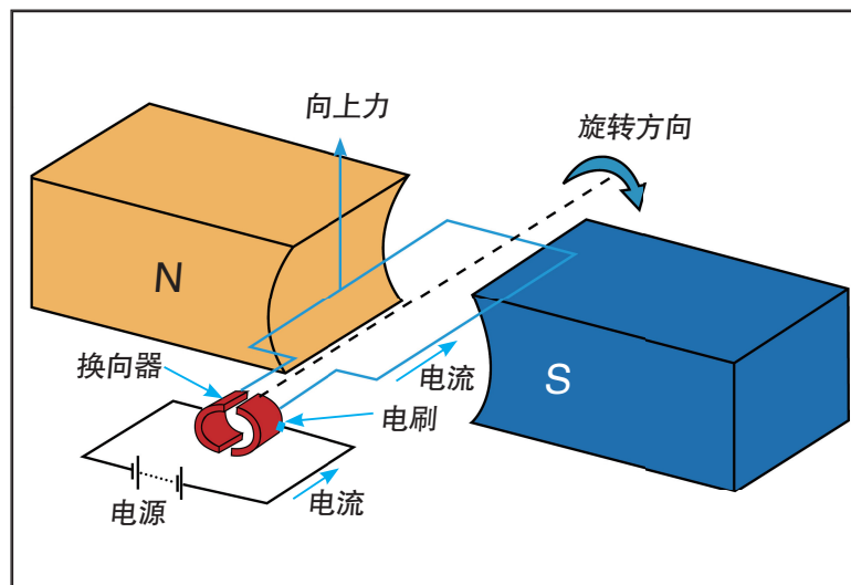
直流电动机原理示意图
