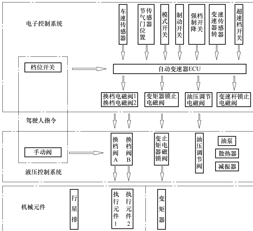
图 1-9 自动变速器换档控制框图
