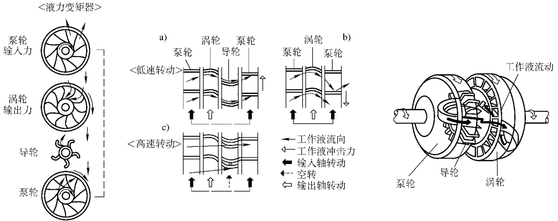
图 1-9 液力变矩器工作时工作液的流向
