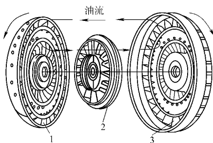
图 1-4 液力变矩器的组成
