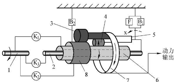
图 1-21 01M 型自动变速器 1 挡工作原理 1—输入轴 2—中间轴 3—长行星轮 4—短行星轮 5—行星架 6—小太阳轮 7—内齿圈 8—大太阳轮
