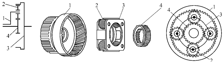
图 1-11 行星轮机构实物图
