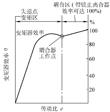
图 1-7 液力变矩器效率特性曲线
