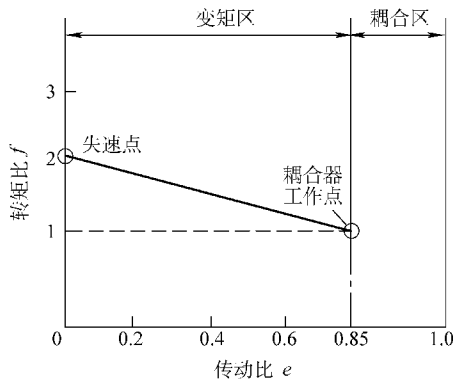
图 1-6 液力变矩器转矩特性曲线
