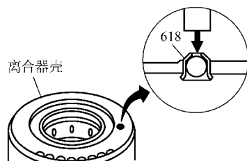
图 1-16 单向球阀的结构
