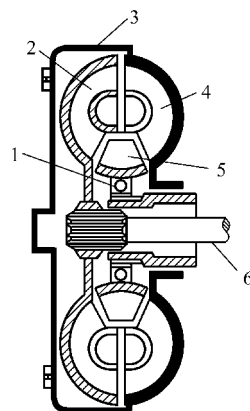
图 1-5 液力变矩器的内部结构
