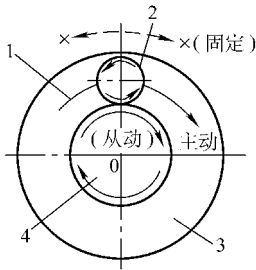
图 1-10 行星轮机构示意图
