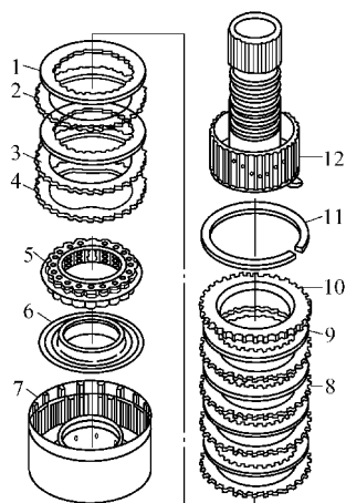
图 1-14 湿式多片离合器分解
