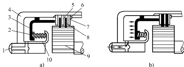
图 1-15 湿式多片离合器的工作原理
