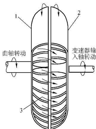
图 1-3 液力耦合器的工作过程
