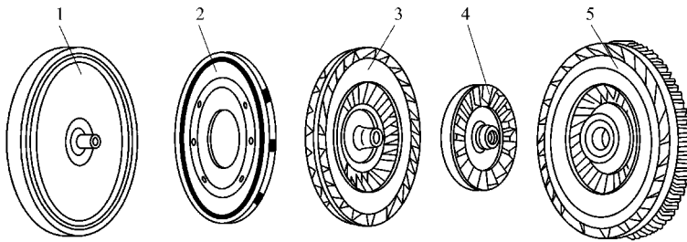
图 1-8 01M 液力变矩器
