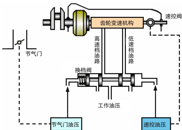
液压控制液力式自动变速器原理图
