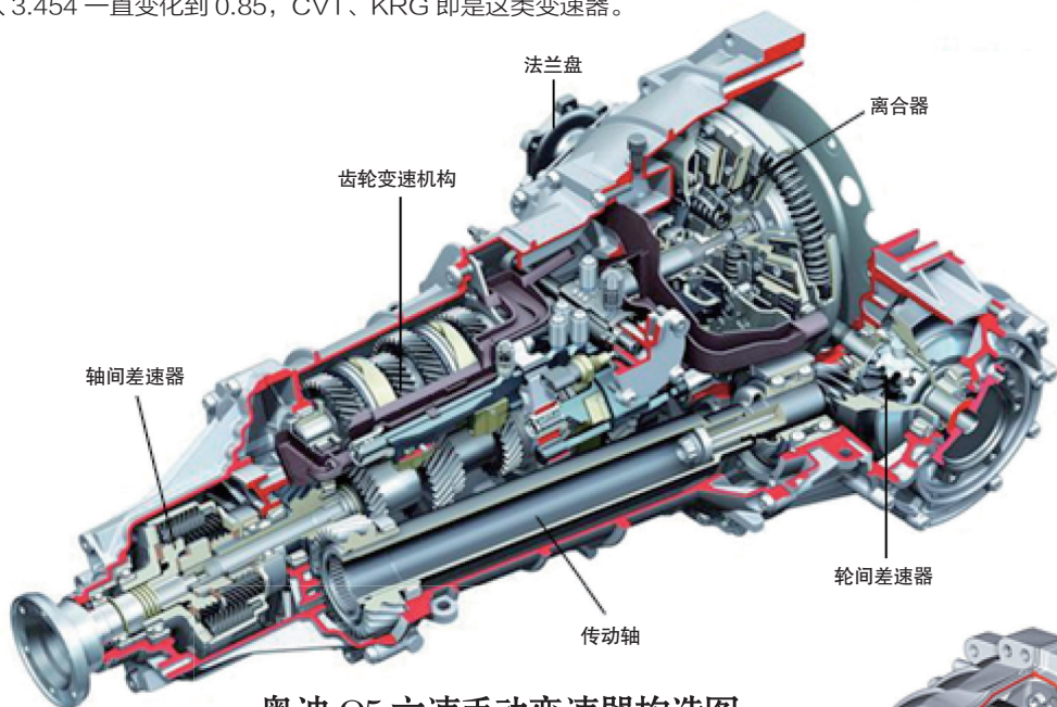
奥迪 Q5 六速手动变速器构造图
