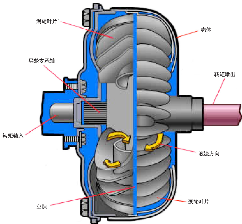
液力传动示意图
