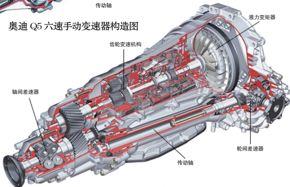
奥迪 09E 自动变速器构造图
