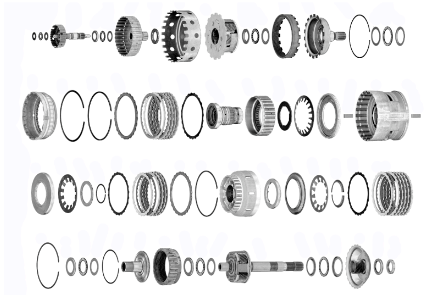
奥迪 01V 变速器部件分解示意图 1
