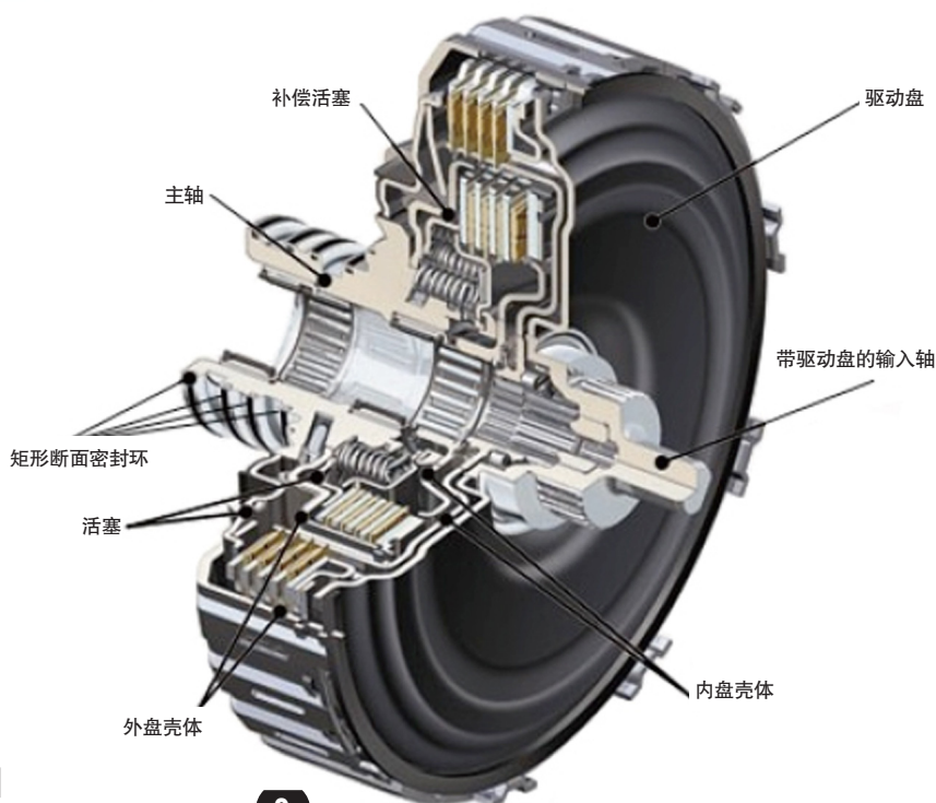
湿式双离合器整体构造图
