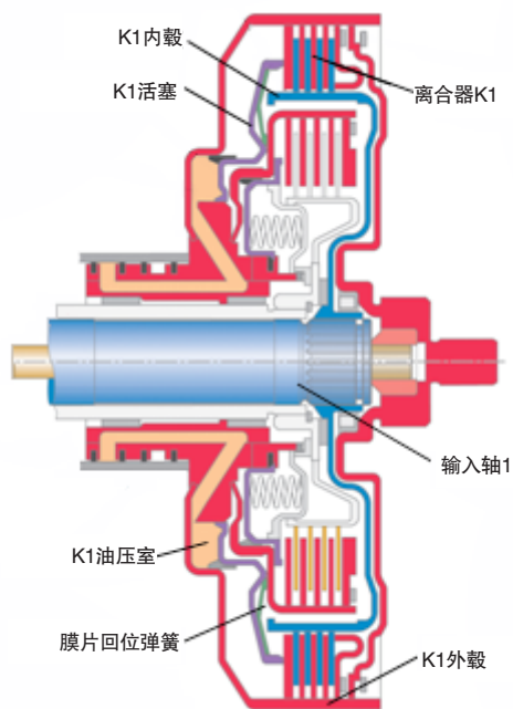
离合器 K1 构造图
