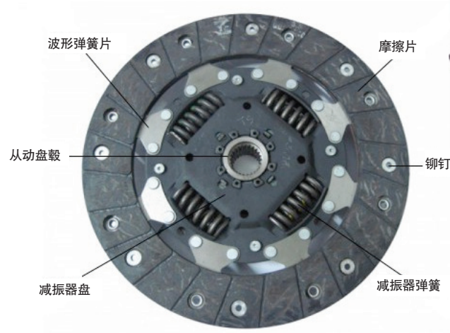
从动盘构造图
