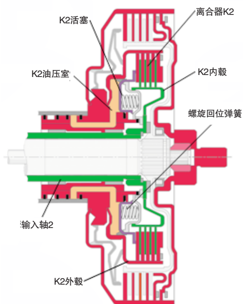
离合器 K2 构造图
