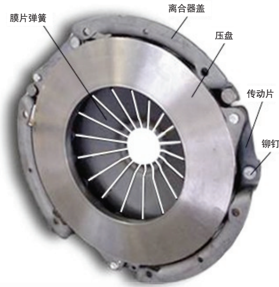
离合器主动部分
