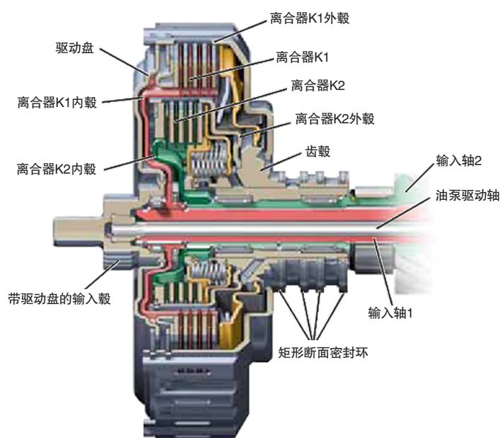
湿式双离合整体构造图
