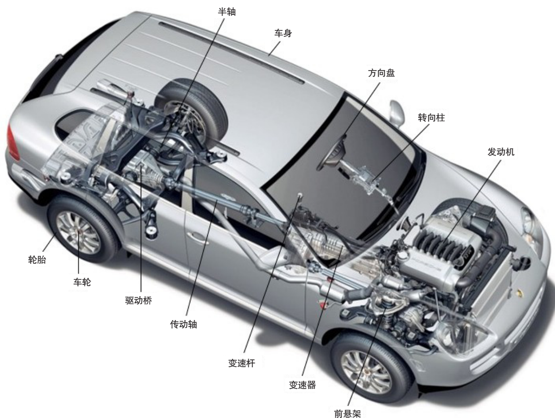
汽车底盘主要部件构造图
