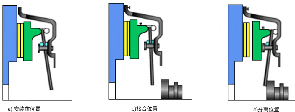
离合器工作原理图
