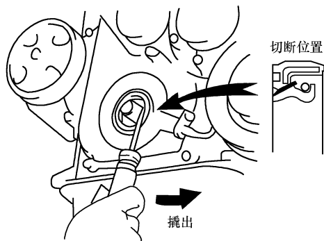
图 1-13 拆出曲轴前油封
