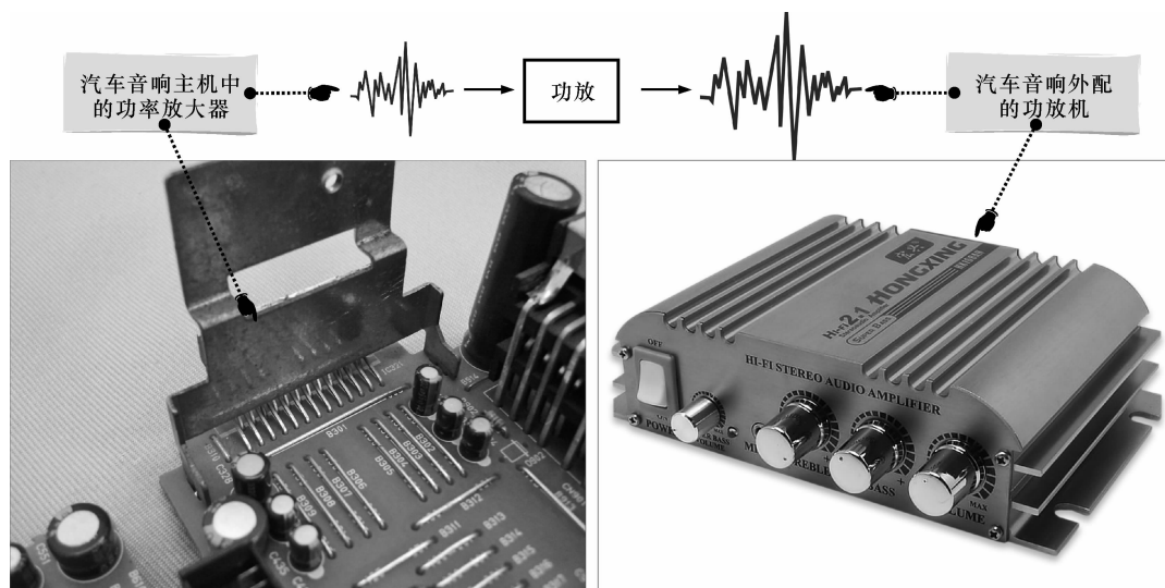
图 1-3 常见功放的实物外形
