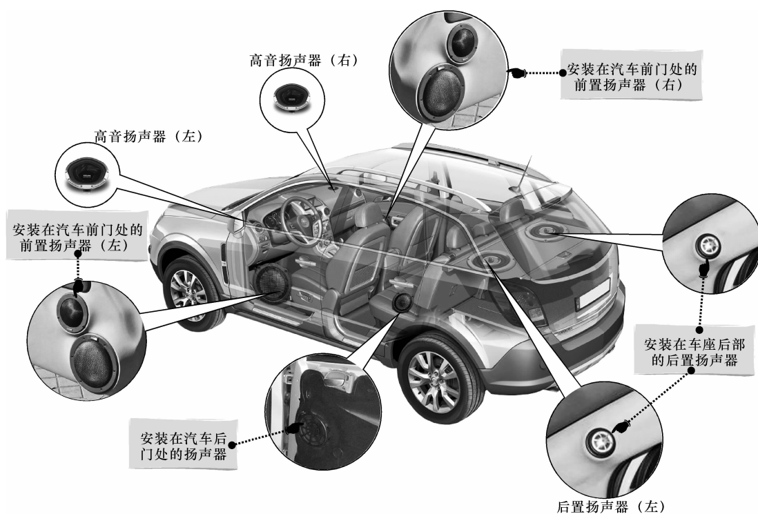
图 1-4 汽车中典型的扬声器及安装位置
