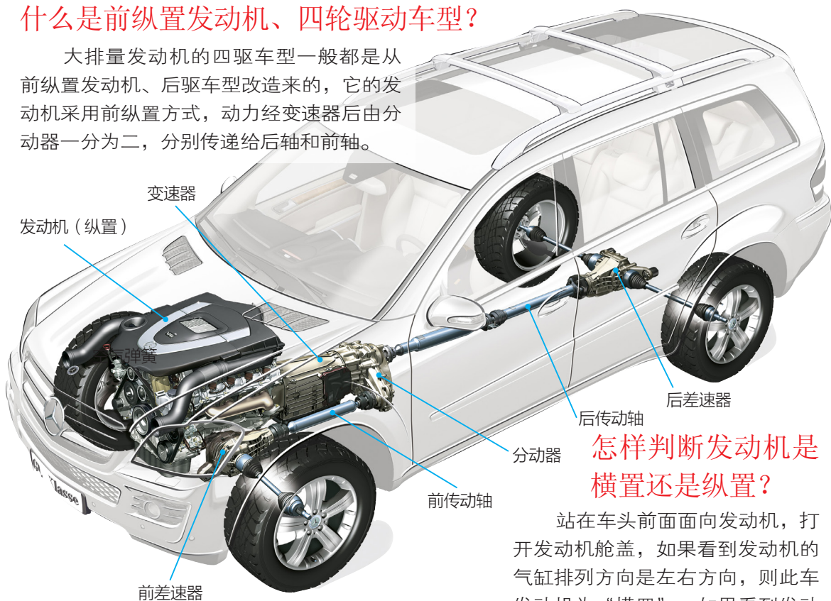
前纵置发动机、四轮驱动车型（奔驰 GL）构造图
