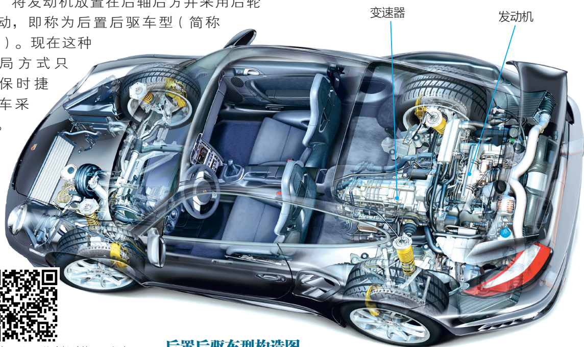
后置后驱车型构造图
