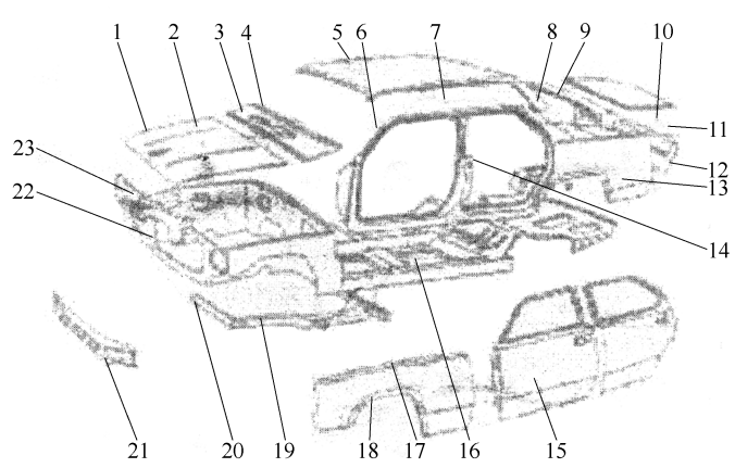
图 1-1 三厢式轿车车身冲压件结构图
