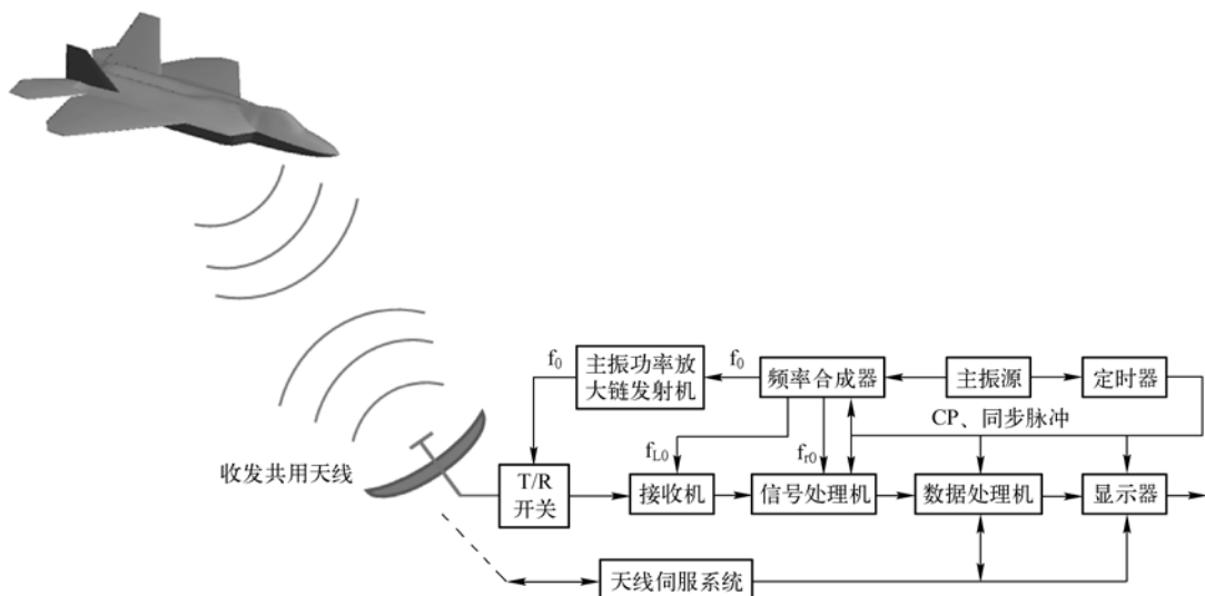
图 1-3 雷达功能框图
