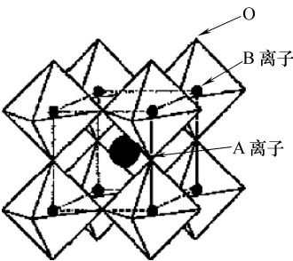
图 1.1 理想的钙钛矿型结构
