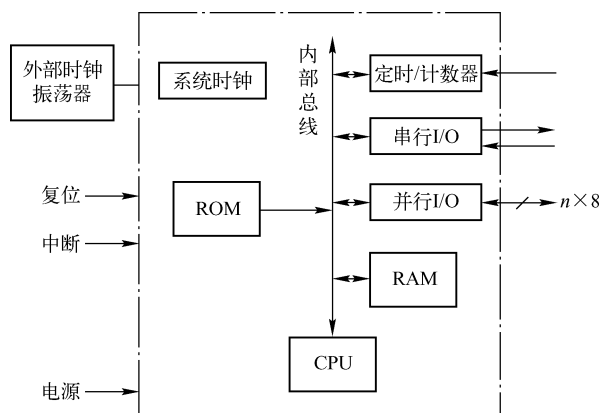
图 1-1 单片机的内部结构框图
