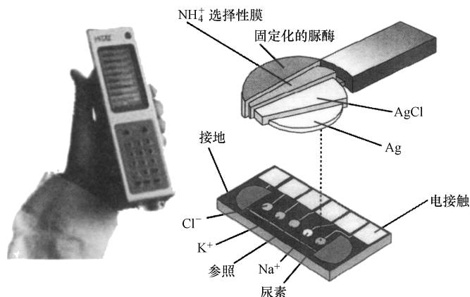
图 1.2 用于监测各种血液中的电解质、气体和代谢物的 i-STAT 多传感器 (www.abottpointofcare.com)
