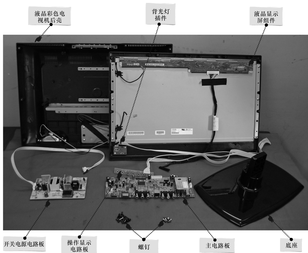
图 1-3 液晶电视机的内部结构
