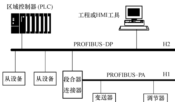
图 1-4 PROFIBUS-PA 系统组成
