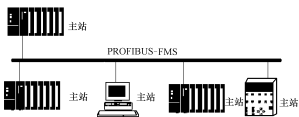
图 1-3 典型的 PROFIBUS-FMS 系统组成
