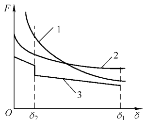
图 1-6 吸力特性与反力特性的配合 1—直流电磁机构吸力特性 2—交流电磁机构吸力特性 3—反力特性
