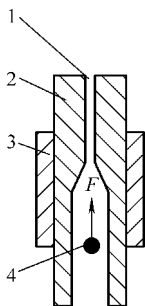
图 1-12 窄缝灭弧示意图 1—纵缝 2—介质 3—磁性夹板 4—电弧
