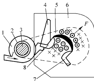
图 1-13 磁吹灭弧示意图 1—吹弧线圈 2—绝缘套筒 3—铁心 4—引弧角 5—导磁夹板 6—灭弧罩 7—动触点 8—静触点
