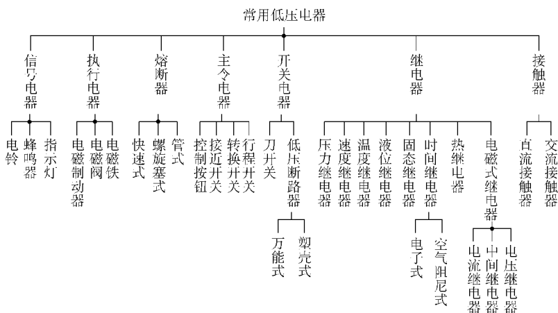
图 1-1 常用低压电器的分类
