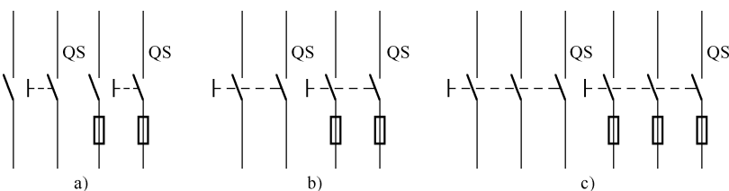
图 1-3 刀开关的图形文字符号 a) 单极 b) 双极 c) 三极
