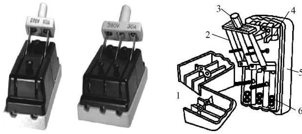
图 1-6 HK2 系列瓷底胶盖刀开关
