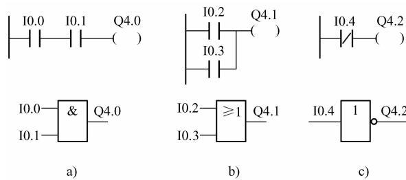
图 1-2 基本逻辑运算
