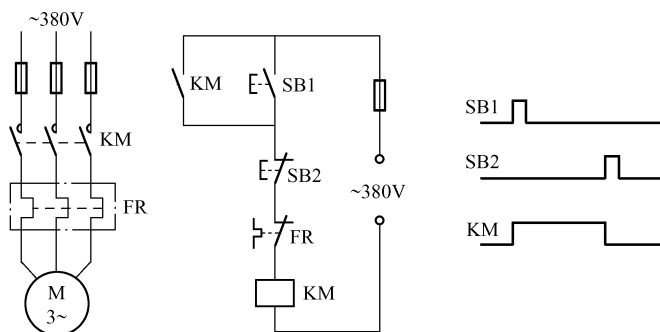
图 1-3 异步电动机控制电路
