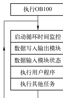
图 1-4 扫描过程
