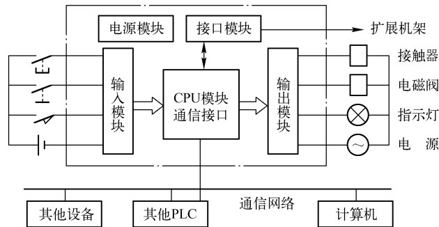
图 1-1 PLC 控制系统示意图
