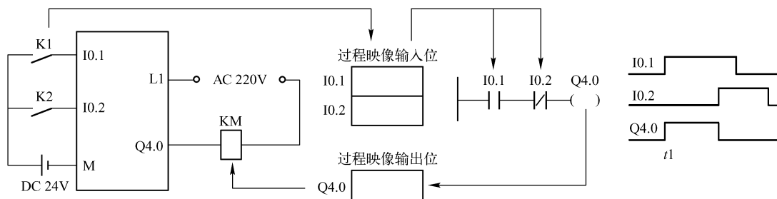
图 1-5 PLC 外部接线图与梯形图
