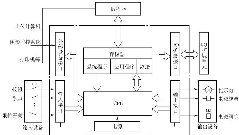
图 1-1 PLC 的典型电路结构图
