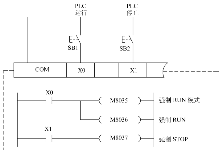
图 1-4 用程序及输入端子控制 PLC RUN/STOP
