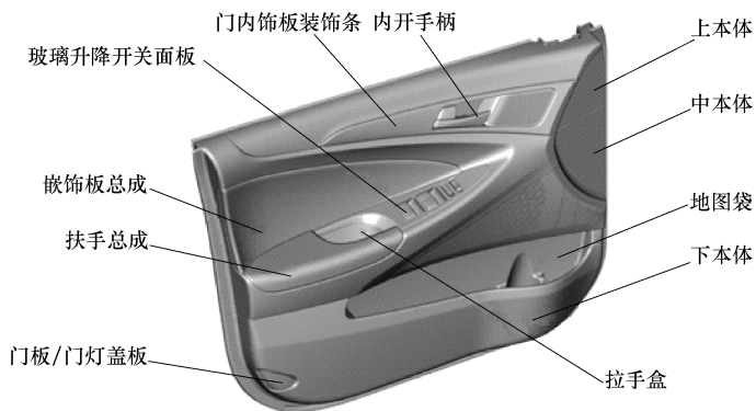
图 1-10 汽车门内饰板系统
