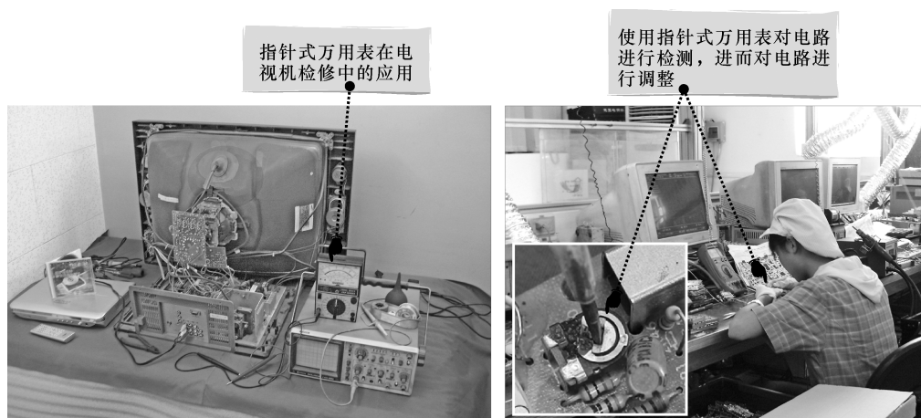
图 1-2 指针式万用表的应用
