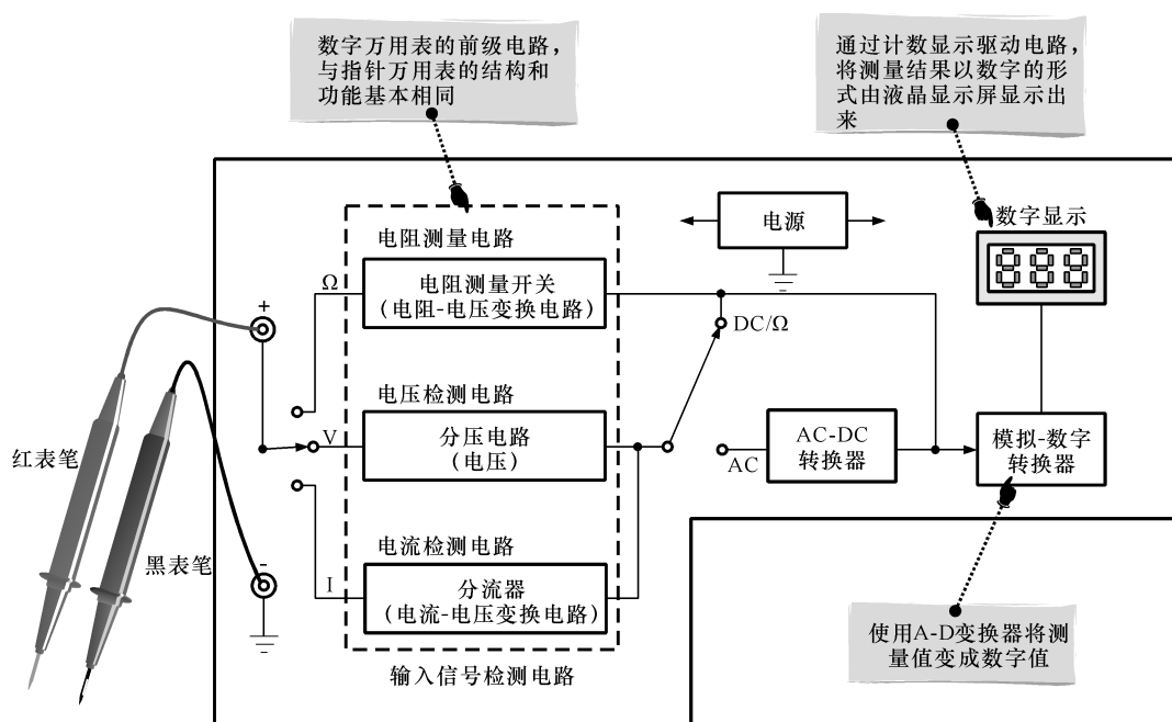
图 1-4 数字式万用表的电路方框图
