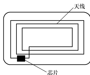
图 2-2 非接触式 IC 卡
