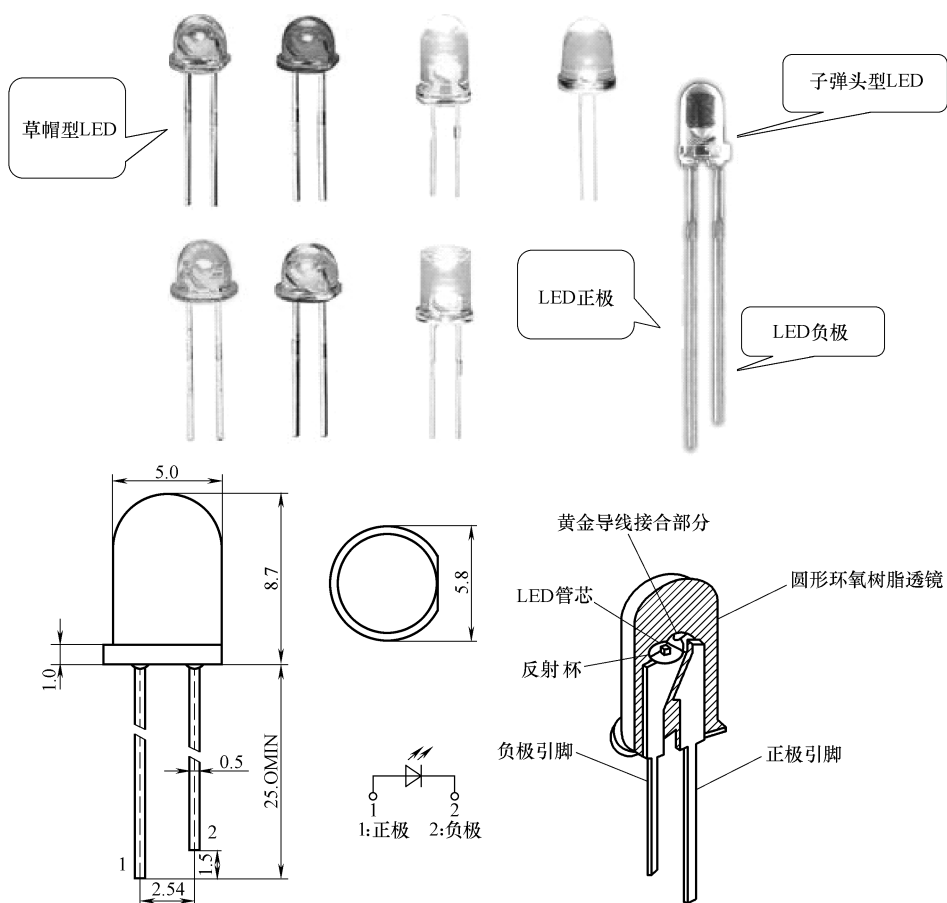
图 1-2 插件型封装外形与结构
